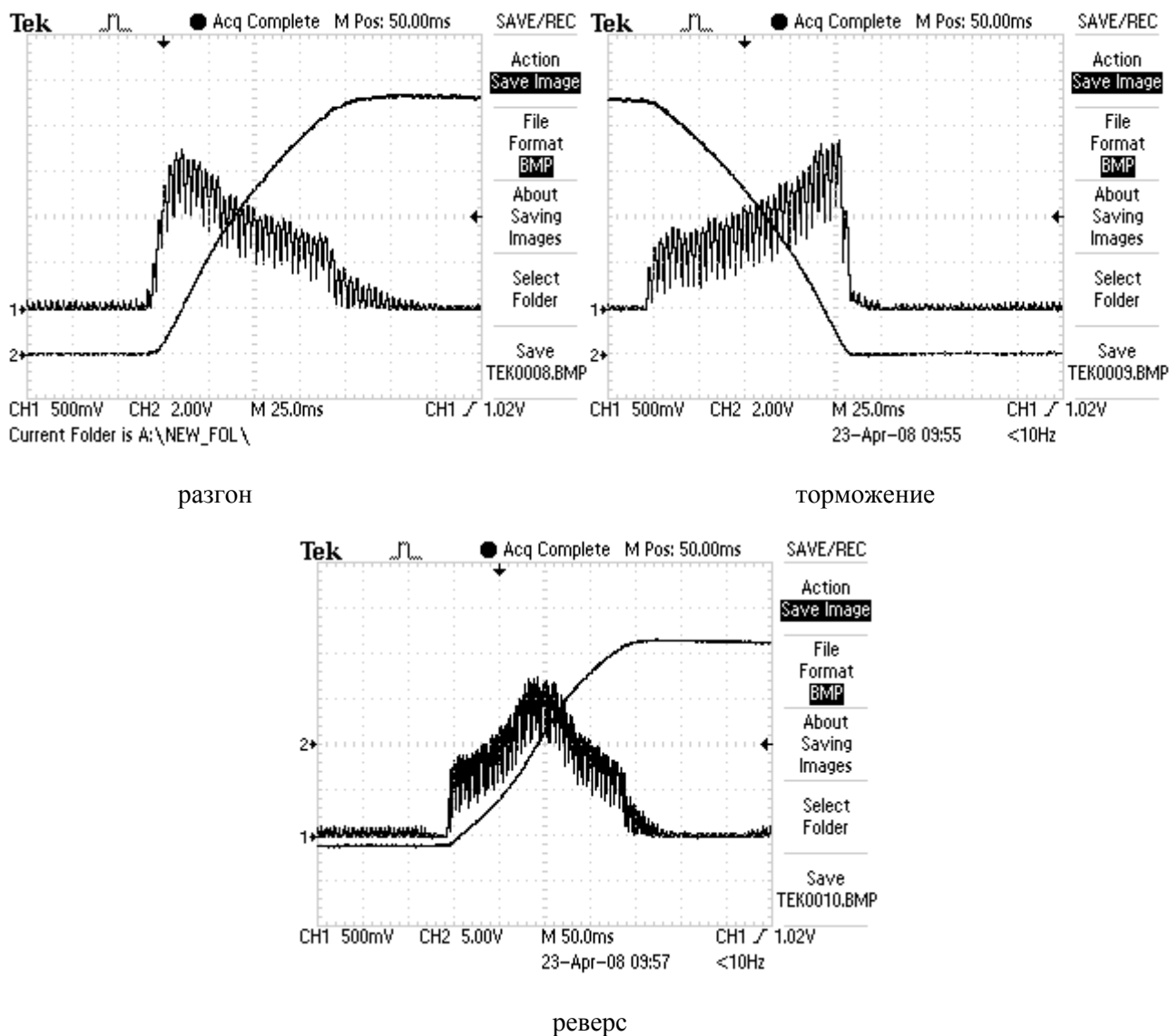
Рисунок 27 Кривые скорости и тока якоря для оптимально настроенного регулятора скорости
