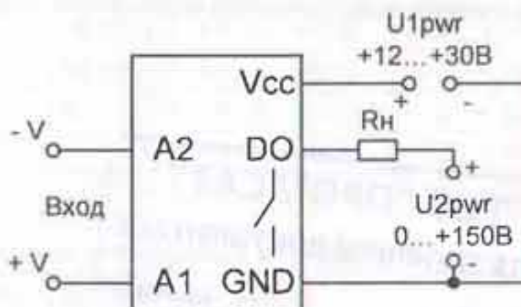
е) питание нагрузки от отдельного источника питания
