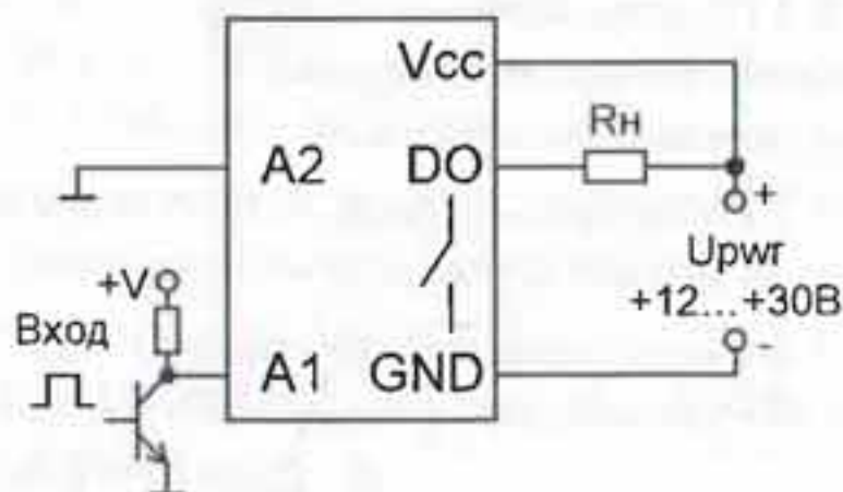
г) выходной транзистор открыт, управление NPN транзистором
