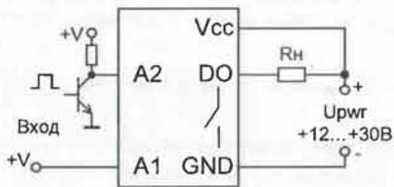
а) выходной транзистор закрыт
