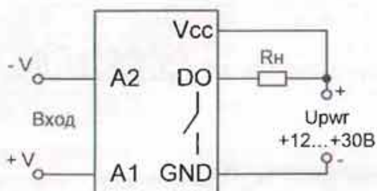
д) питание реле и нагрузки от источника питания 12...30В
