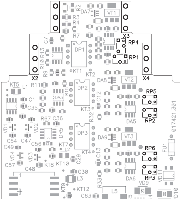
Рис. 10.2 Расположение регулировок на плате растроителя
