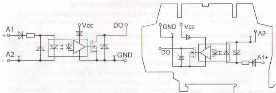
Рис. 4.1 Функциональная схема модуля гальванической развязки
