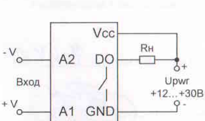
д) питание модуля и нагрузки от источника питания 12...30В
