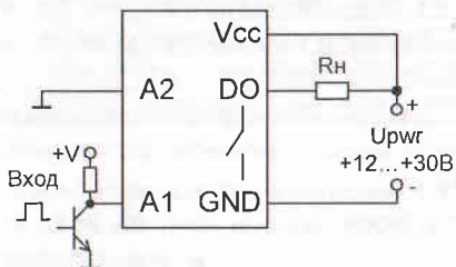
г) выходной транзистор открыт, управление NPN транзистором
