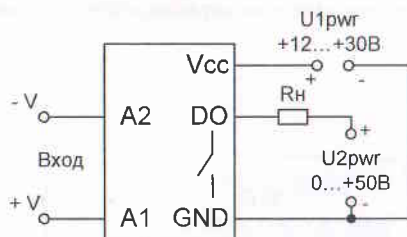
е) питание нагрузки от отдельного источника питания
