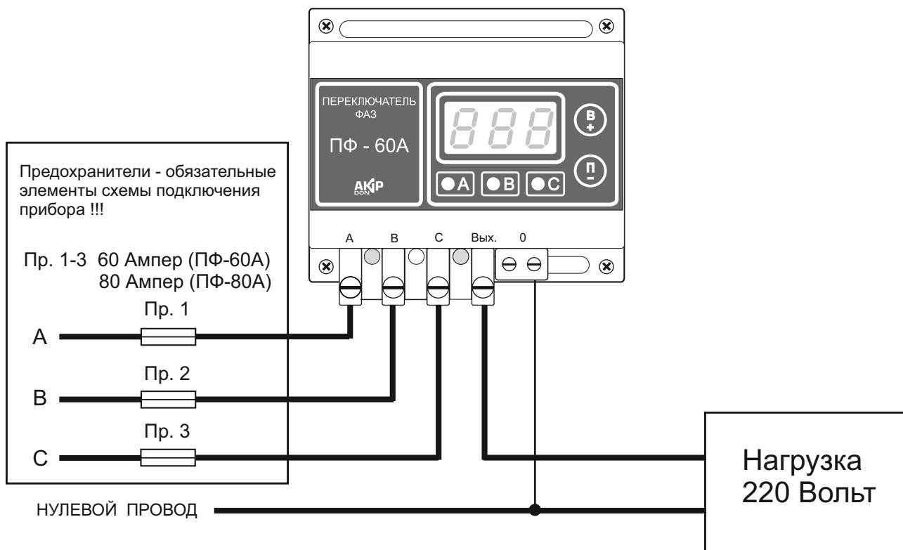
Рис. 2. Схема подключения приборов ПФ-60А, ПФ-80А к 3х фазной электросети.
