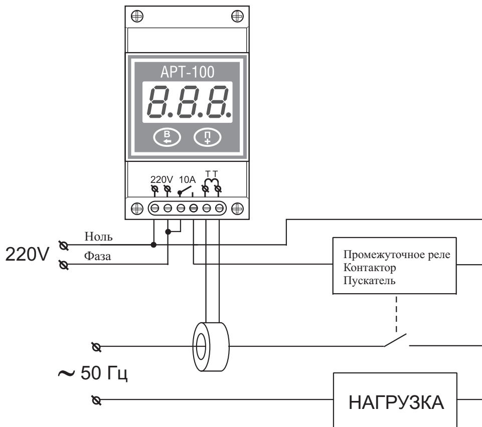
Рис.1 Вариант подключения прибора.
