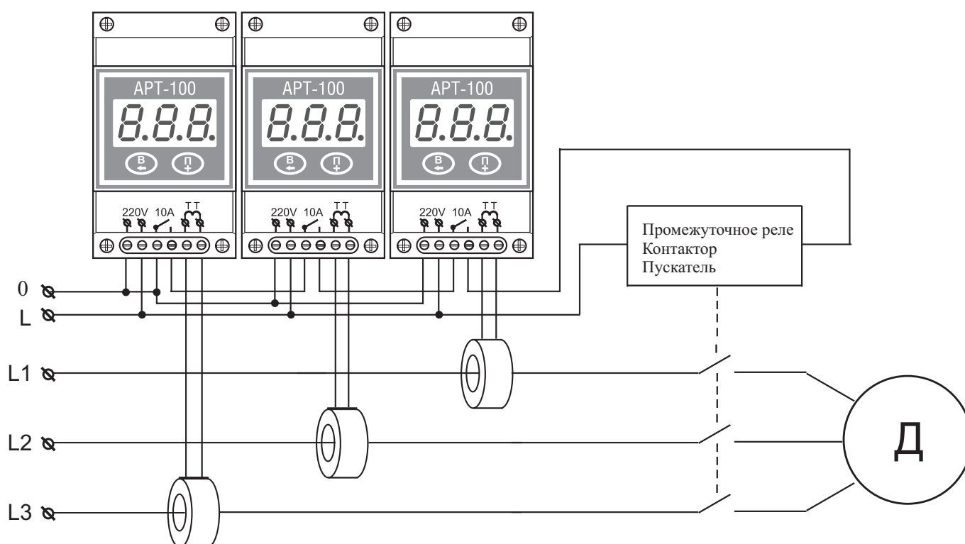
Рис.2 Вариант защиты по току трехфазного потребителя.
