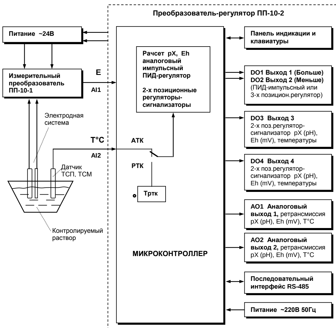
Рисунок 5.2. Структурная схема микропроцессорного преобразователь-регулятора потенциометрического ПП-10-2, в комплекте с измерительным преобразователем ПП-10-1
