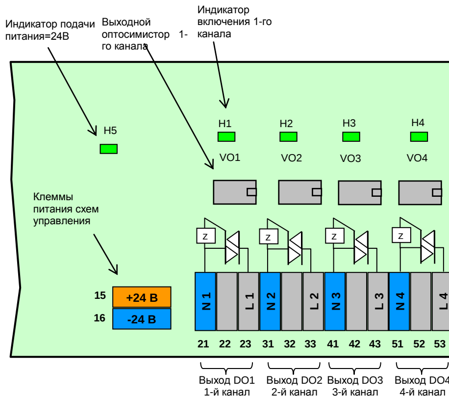
Рисунок Б.18 - Подключение дискретных нагрузок с помощью КБЗ-28С-11
