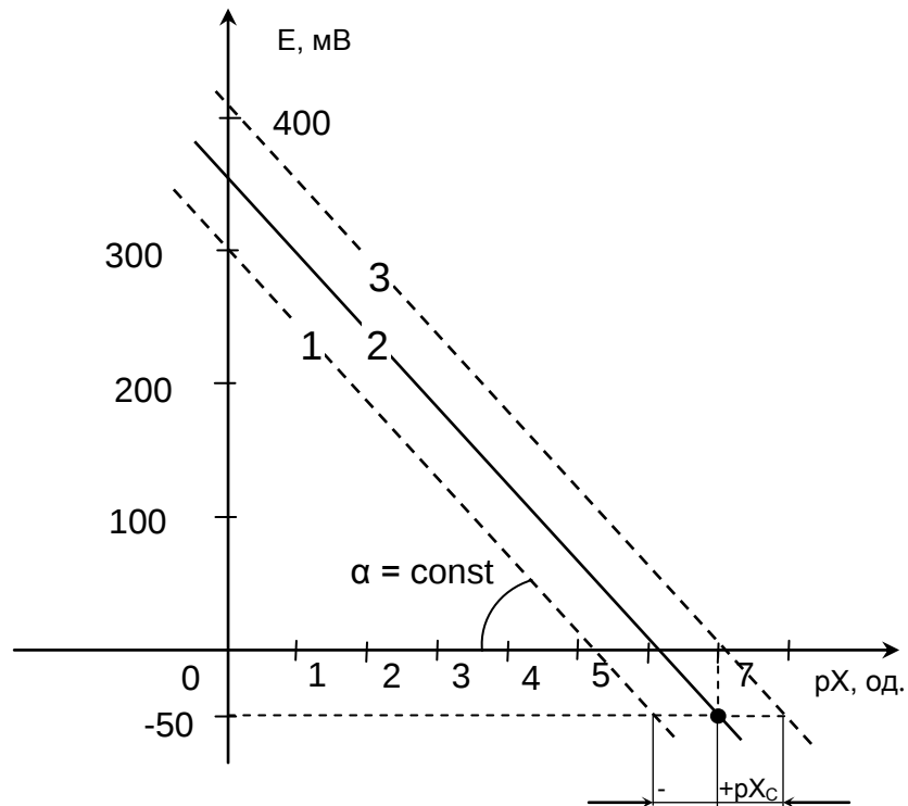
Рисунок 5.5. Коррекция смещения pX_{СМ} электродной характеристики.
