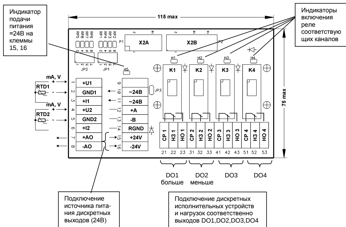
Рисунок Б.16 - Подключение дискретных нагрузок с помощью КБЗ-28Р-11
