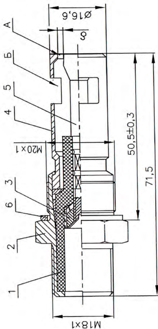
Свеча плазмоструйная СП-1-2
