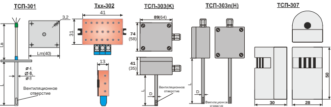
Рисунок 6 - Группа 3. Преобразователи воздушные
