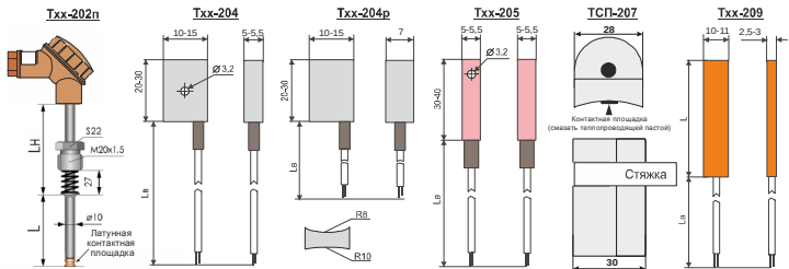
Рисунок 5 - Группа 2. Преобразователи поверхностные
