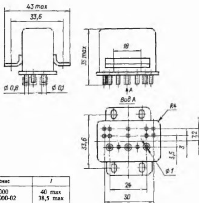
Рис. 2-194. Конструктивные данные реле РПА14
