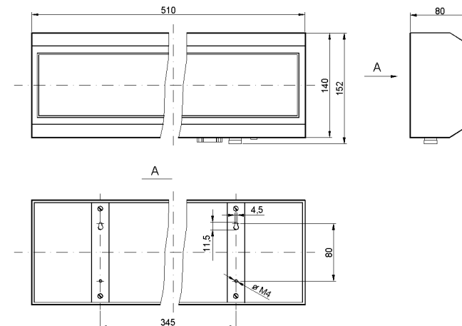
Габаритные и установочные размеры панели K920-01
